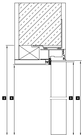
Sección vertical con hoja de puerta sin galce (hoja enrasada)
