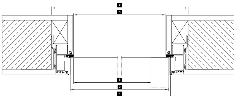
Sección horizontal con hoja de puerta sin galce (hoja enrasada)
