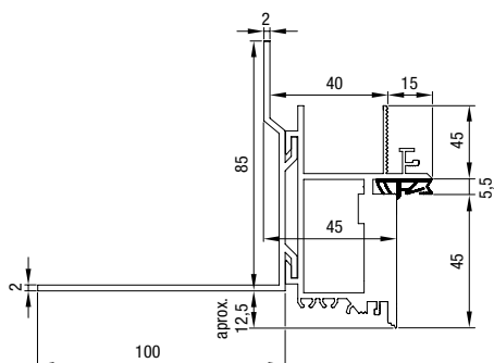
Dimensiones cerco (marco oculto)
