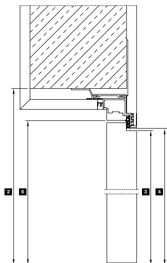
Sección vertical con hoja de puerta que se abre al revés
