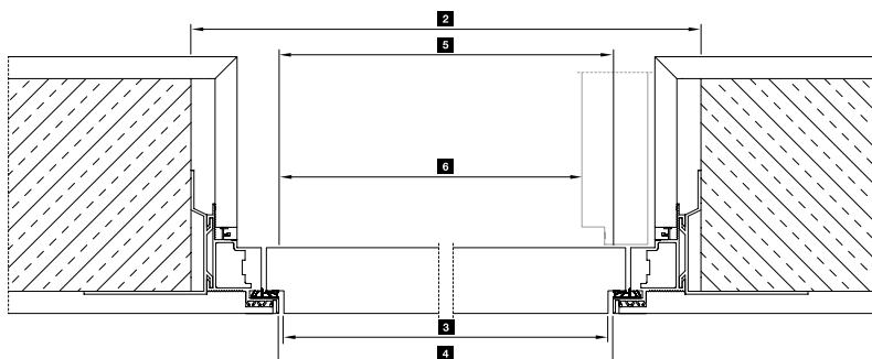
Sección horizontal con hoja de puerta que se abre al revés
